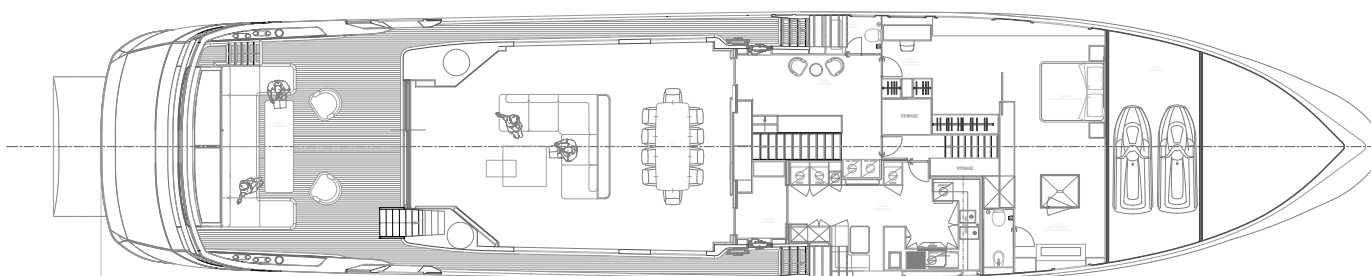
MAINDECK
