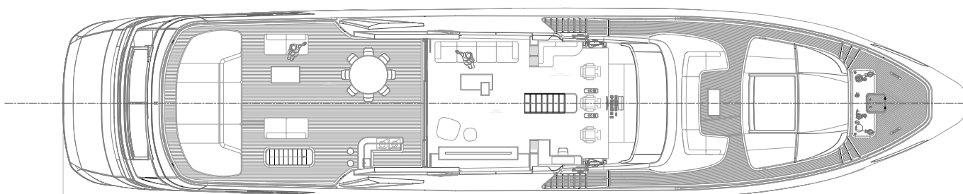
UPPERDECK
